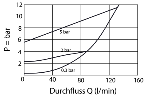
Typischer Druckabfall
