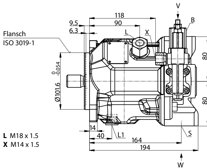
Anschlussplatte 12
