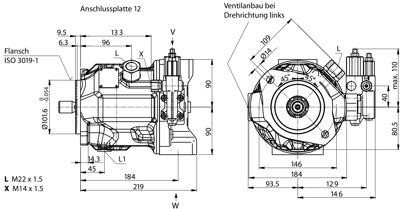
Teilansicht V
