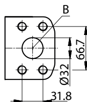
Teilansicht V
