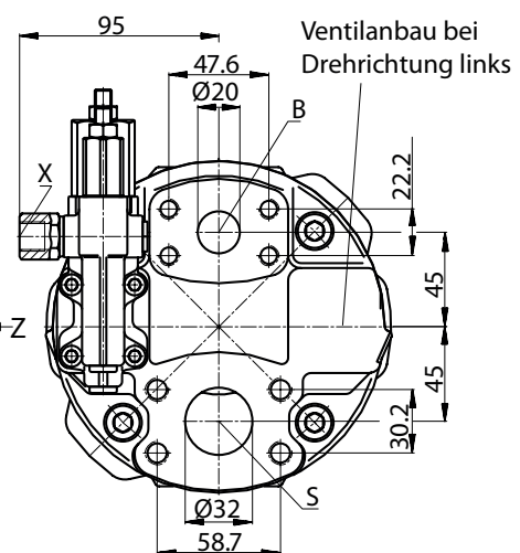
Ansicht Z
