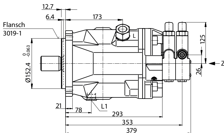
Anschlussplatte 11
