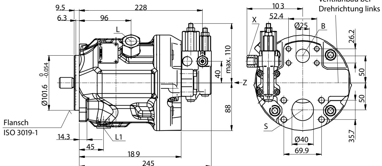
Ansicht Z
