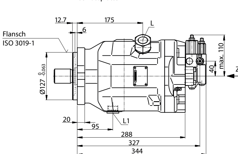
Anschlussplatte 11
