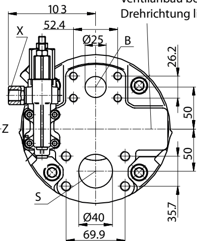
Ansicht Z
