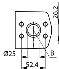
Teilansicht V
