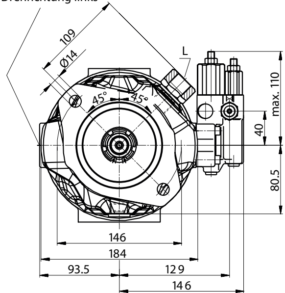
Ventilanbau bei Drehrichtung links
