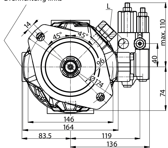
Ventilanbau bei Drehrichtung links
