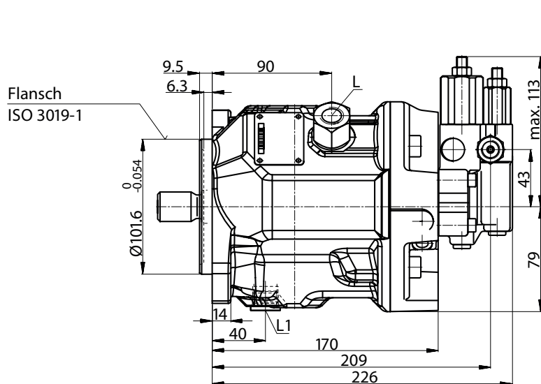
Anschlussplatte 11
