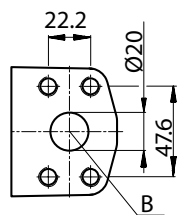
Teilansicht V
