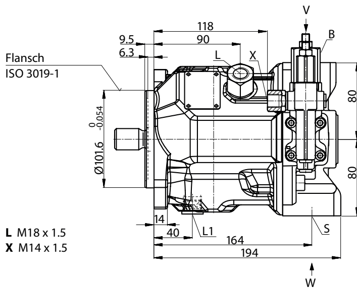
Anschlussplatte 12
