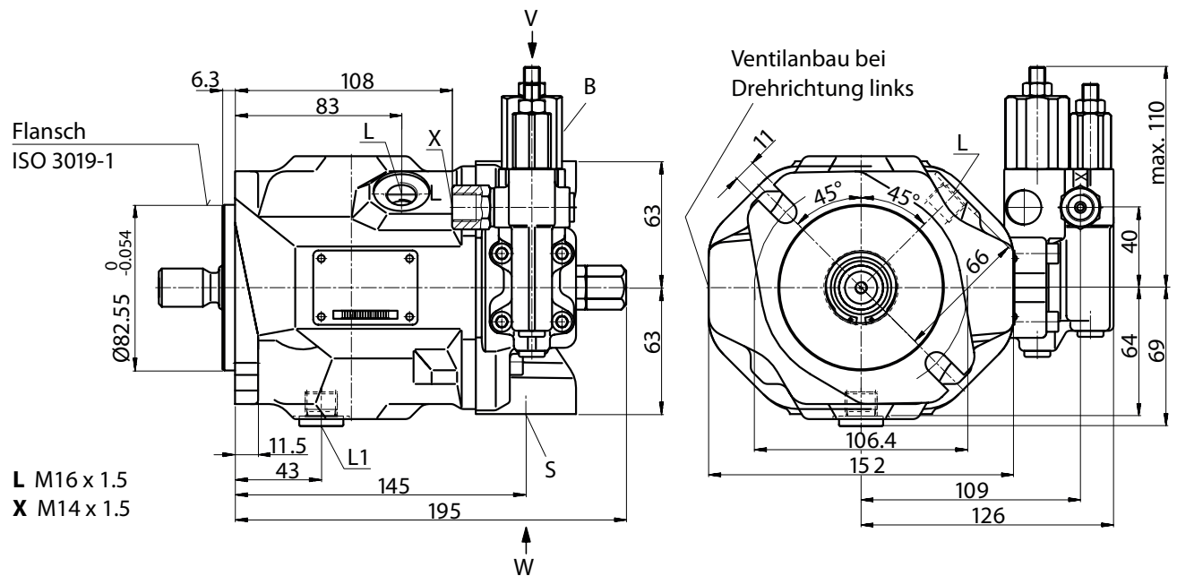
Ansicht V
