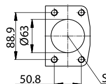
Teilansicht W
