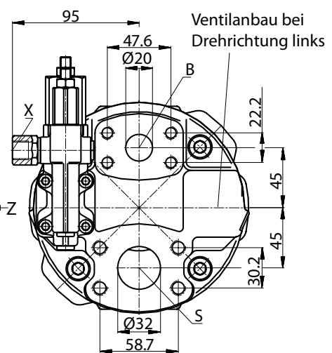
Ansicht Z
