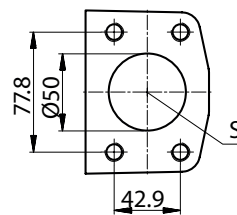
Teilansicht W
