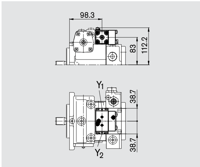
Elektrische Zweipunktverstellung mit Schaltmagnet, EZ
