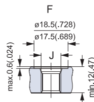
F: UNF Leckölanschluss J: 7 / 16 - 20 UNF O-Ring-boss port
