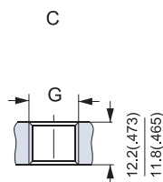
C: BSPP-Leckölanschluss G: ISO 228/1 - G 1 / 4
